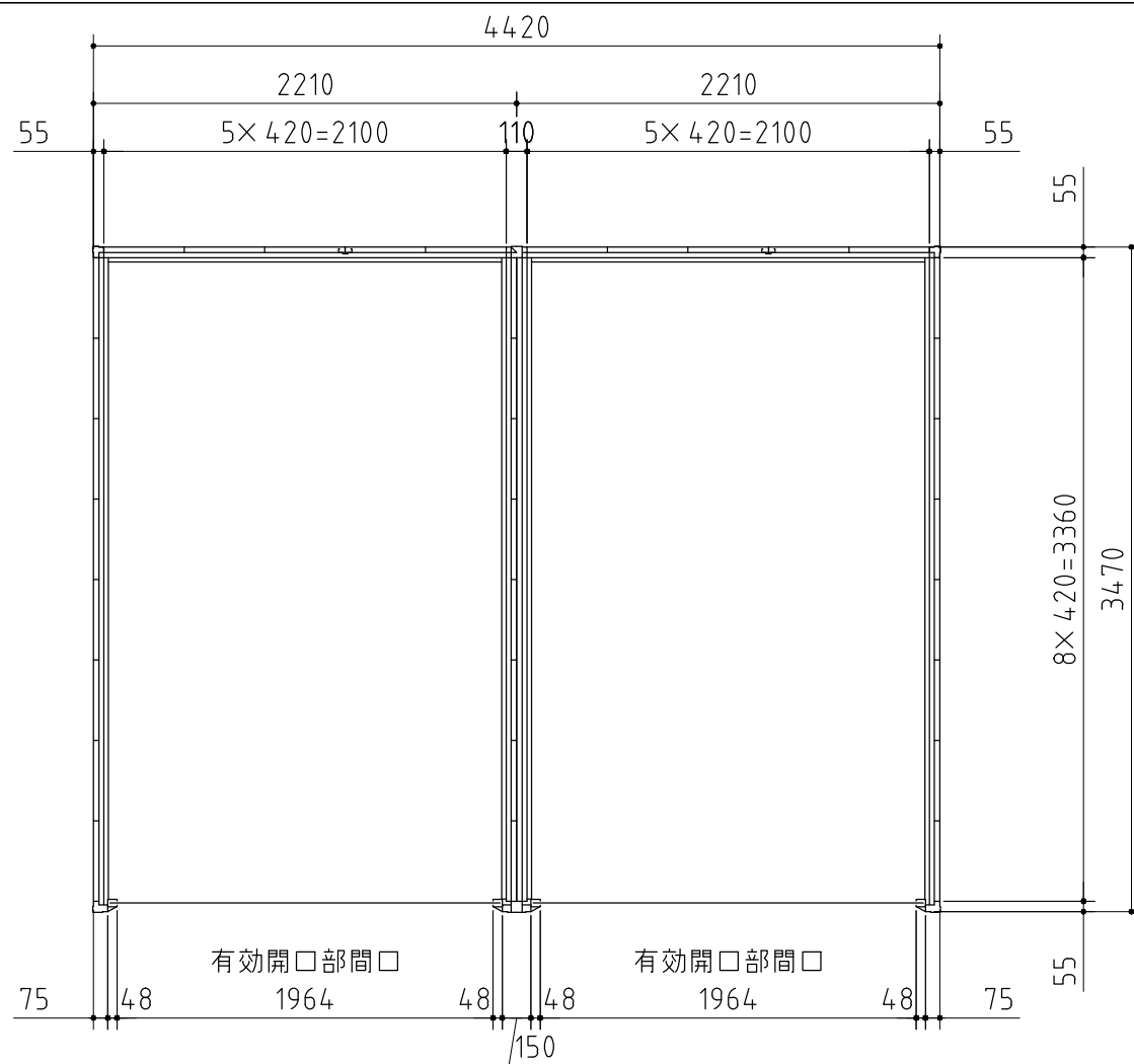
平面図
